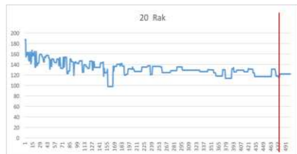
Gambar 10. Konvergensi Harmony Search
