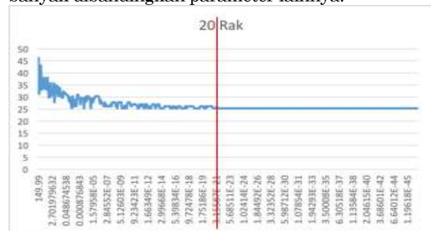
Gambar 9. Konvergensi Simulated Annealing
