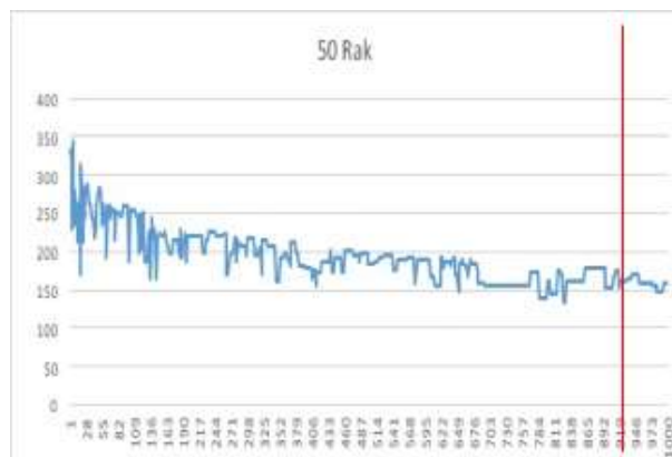
Gambar 6. Konvergensi Harmony Search
